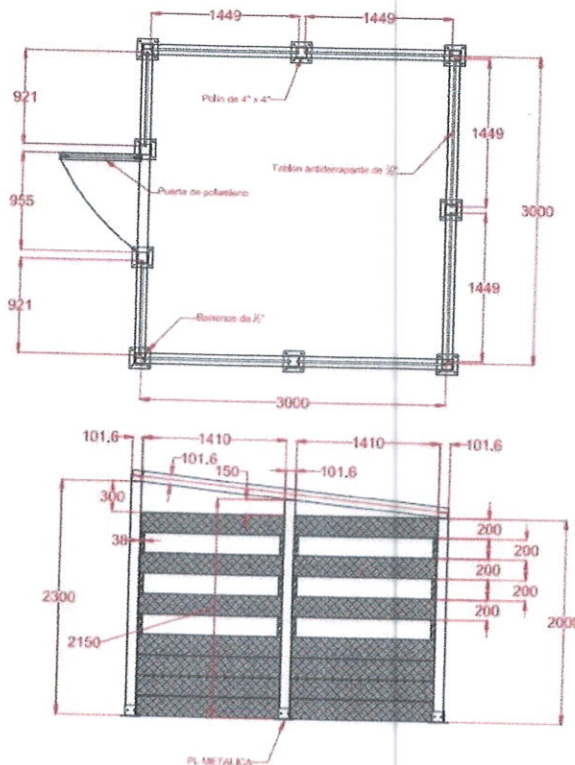
Propuesta inicial de Plano del Centro de Acopio Primario
